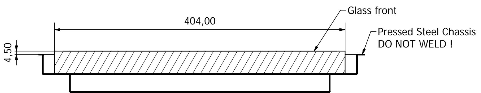
A-A ( 1 : 3 )
